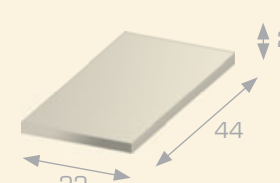
Deska 0300 440 220 / A Hmotnost: 3,8 kg Jednotková hodnota: 3,0
